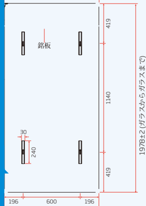
背面図 (横置き)
