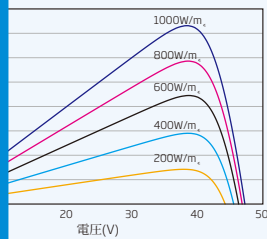
72セル (365W) の P-V 曲線
