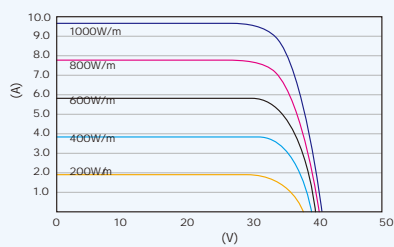
PVモジュール (305W) の I-V 曲線
